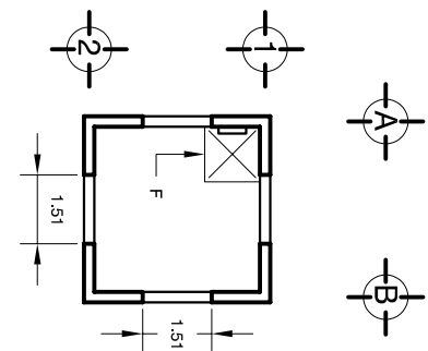
PLANTA CAMPANARIO
