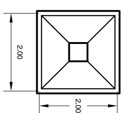
PLANTA AZOTEA
