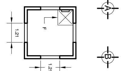
PLANTA CAMPANARIO
