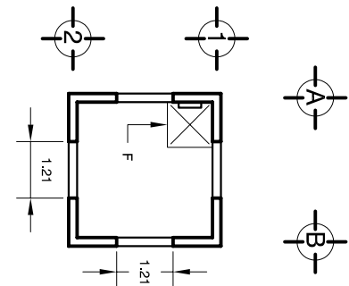
PLANTA CAMPANARIO
