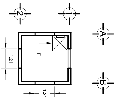
PLANTA CAMPANARIO
