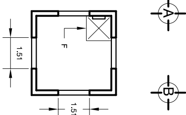
PLANTA CAMPANARIO
